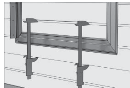
Выверните полосы на нижнем сегменте калитки с полосами на полотне ворот.
